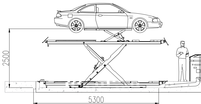
MẶT BẰNG LẮP THIẾT BỊ CẦU NÂNG CẮT KÉO HL-52F
