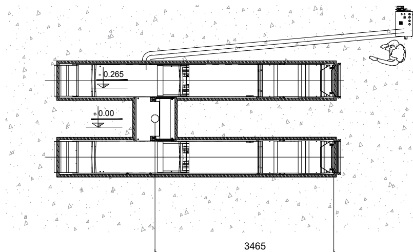
MẶT BẰNG LẮP THIẾT BỊ CẦU NÂNG CẮT KÉO HL-52F
